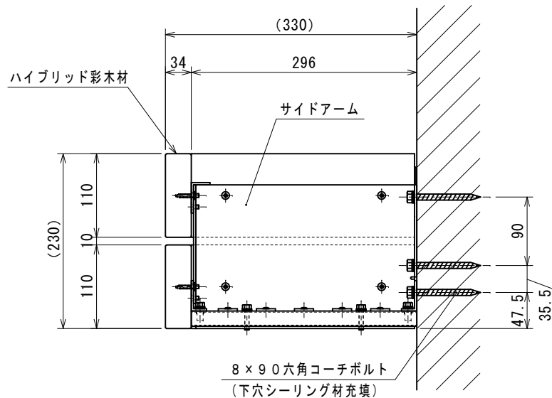
断面詳細 (1:5)
