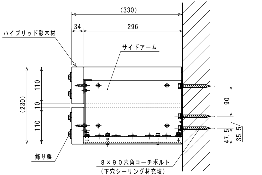
断面詳細 (1:5)
