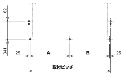
コーチスクリュー下穴位置図
