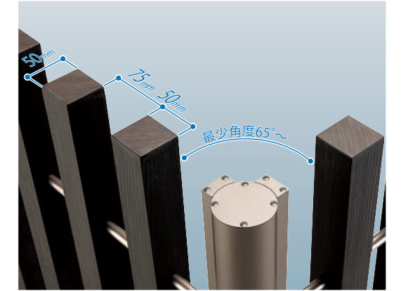
50×50縦格子タイプの上端部は木口模様があります。
