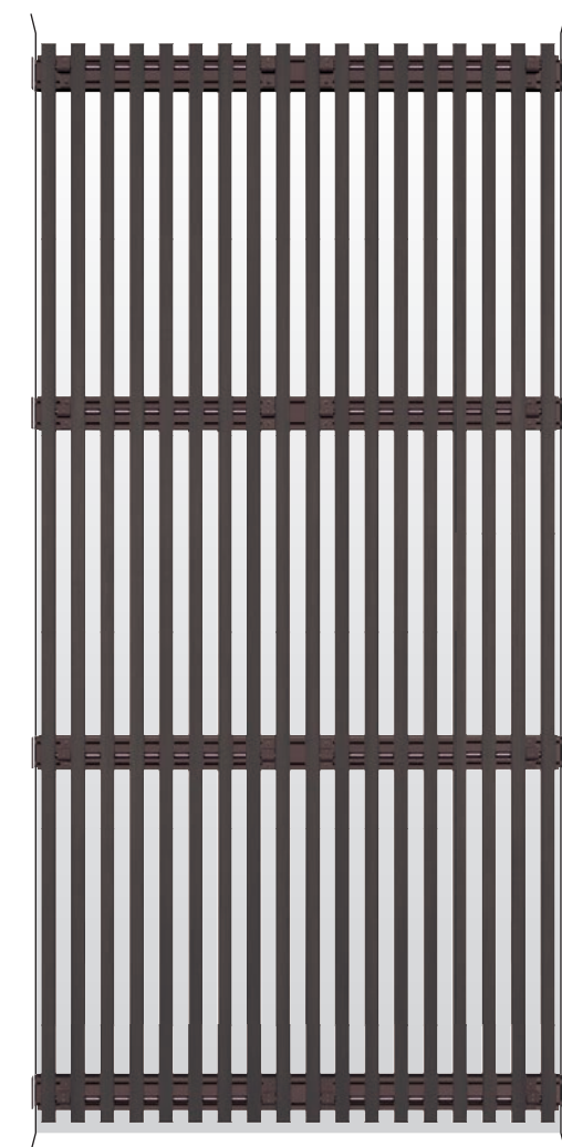
スクリーンの連続部は34mmの隙間を開けて施工します。スクリーンの横棧は連結しません。 40mm×80mm角のアルミ製梁材を開口部に取付けてからスクリーンを連続施工します。
