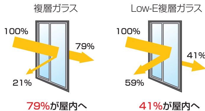
<ガラスの日射侵入率> ※(社)日本サッシ協会
