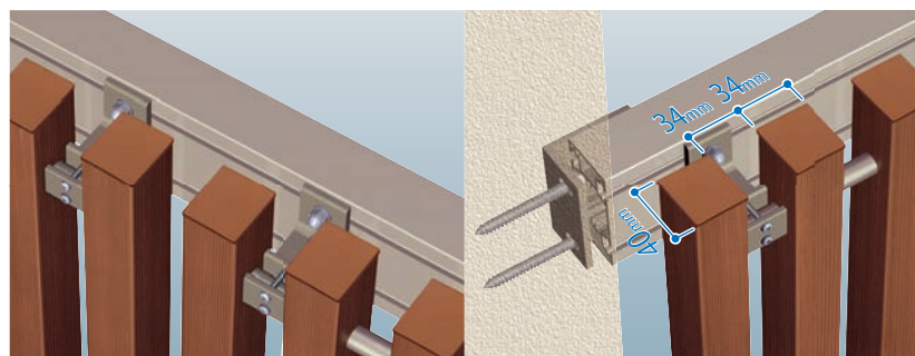
スクリーンの連続部は34mmの隙間を開けて施工します。スクリーンの横棧は連結しません。 40mm×80mm角のアルミ製梁材を開口部に取付けてからスクリーンを連続施工します。
