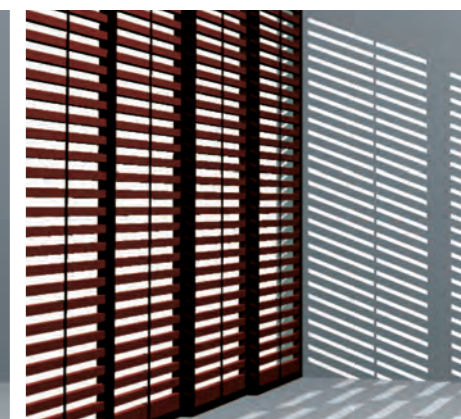
冬至の陽射しのシミュレーション
