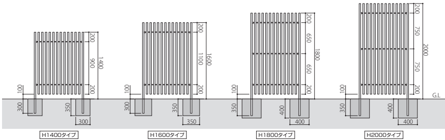
34×40縦格子タイプの上端部は樹脂キャップです。
