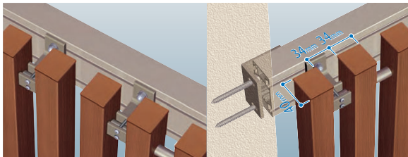
スクリーンの接続部は34mmの隙間を開けて施工します。スクリーンの横棧は連結しません。 40mm×80mm角のアルミ製梁材を開口部に取付けてからスクリーンを連続施工します。
