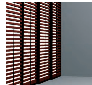
夏夏の陽射しのシミュレーション
