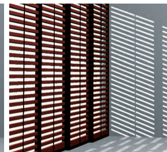
冬冬の陽射しのシミュレーション
