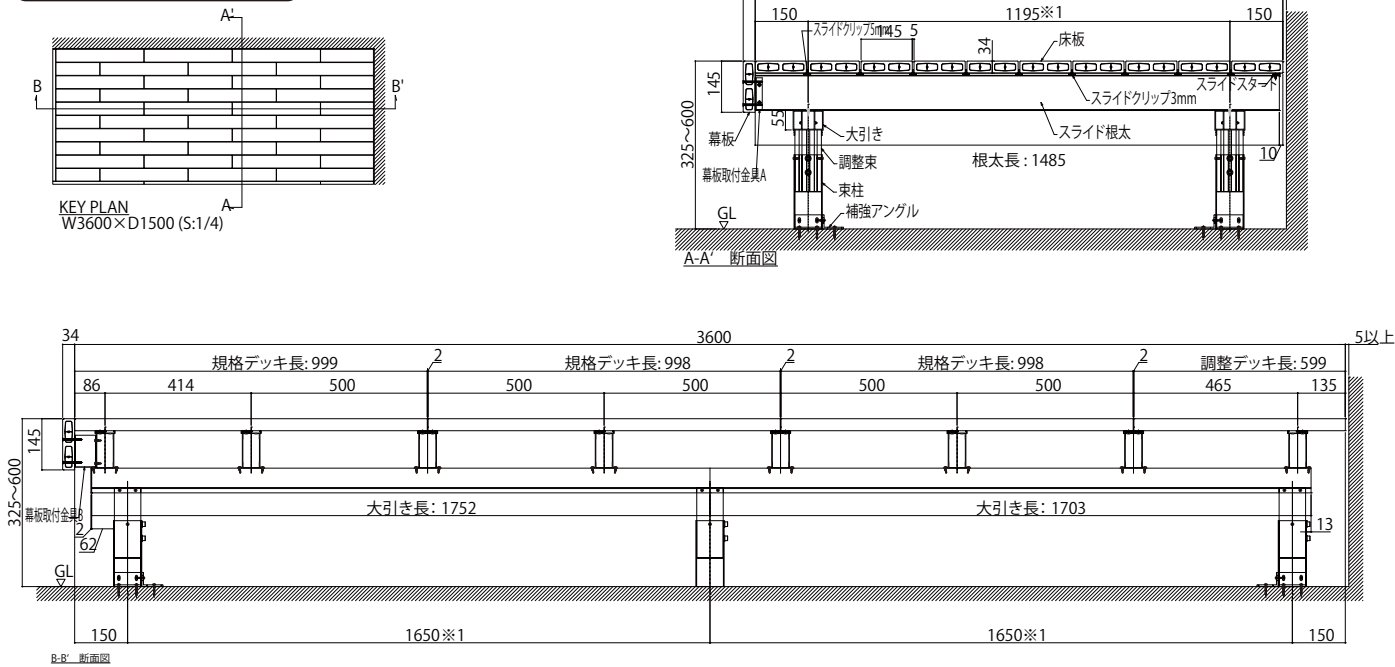
彩木ガーデンデッキ・断面図
