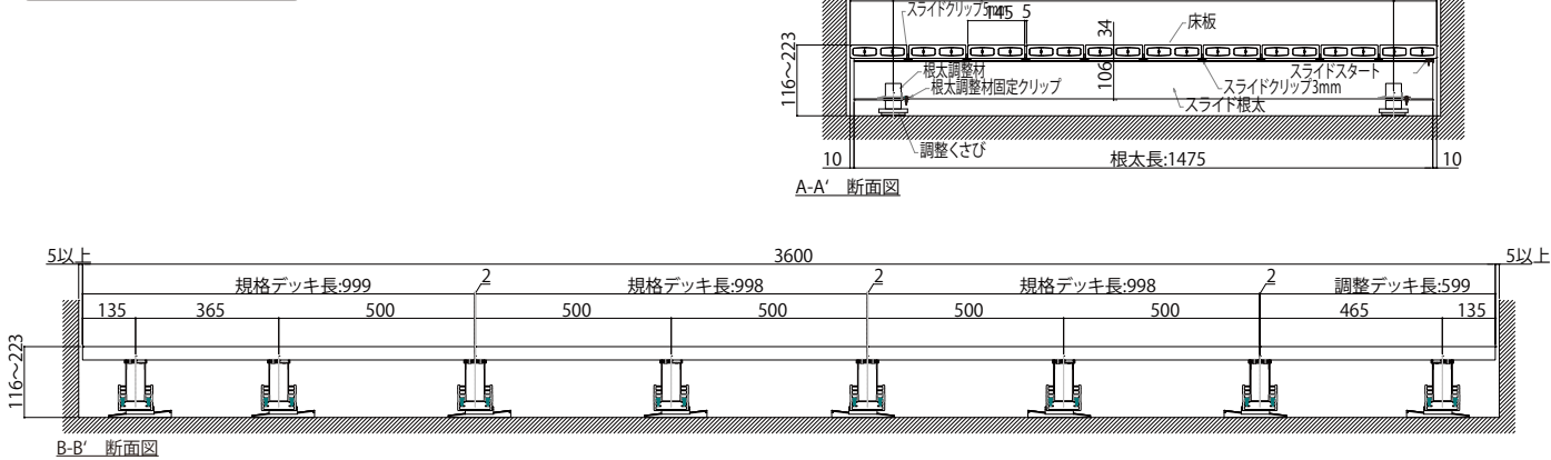
彩木ルーフデッキ・断面図
