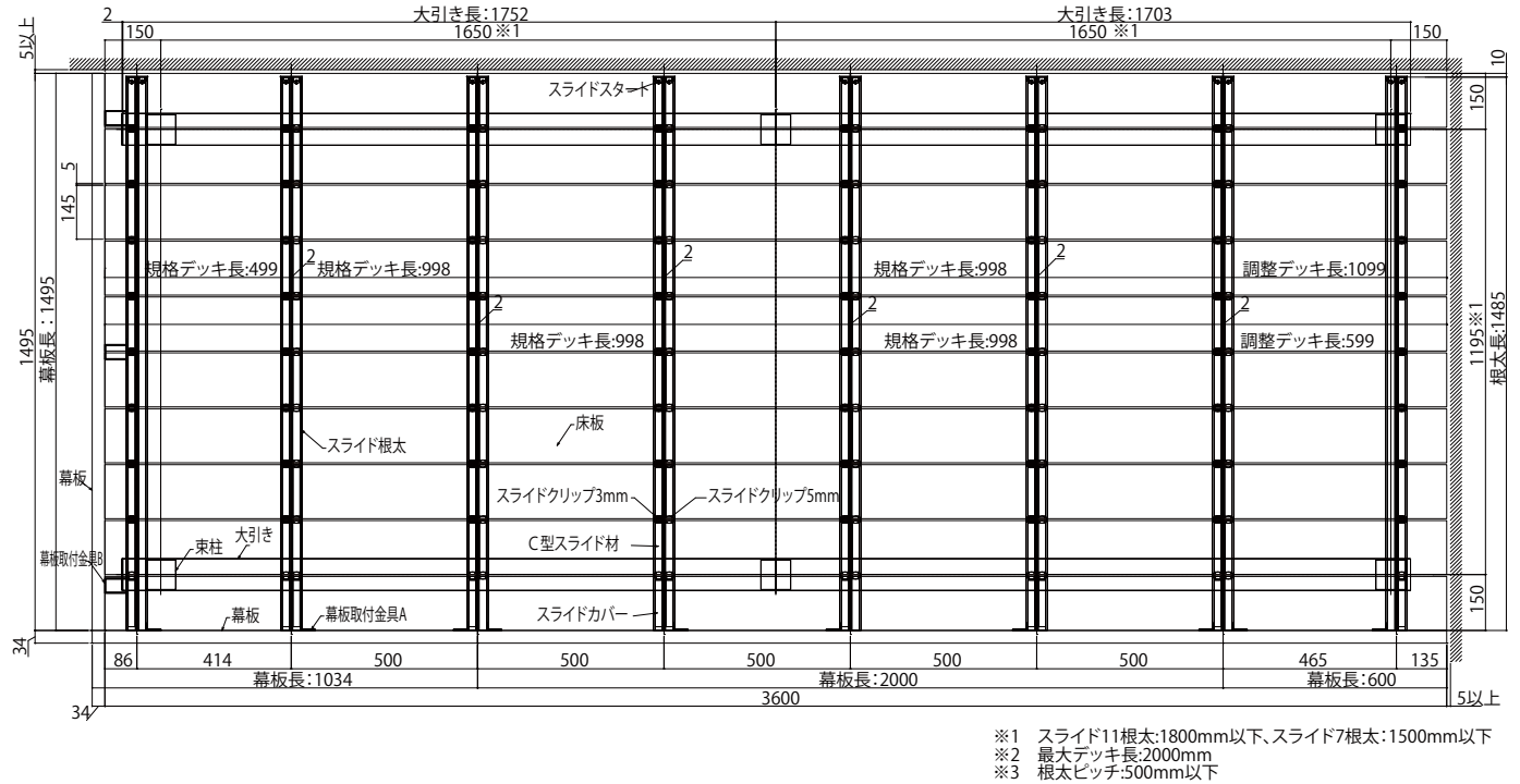
彩木デッキ平面図
