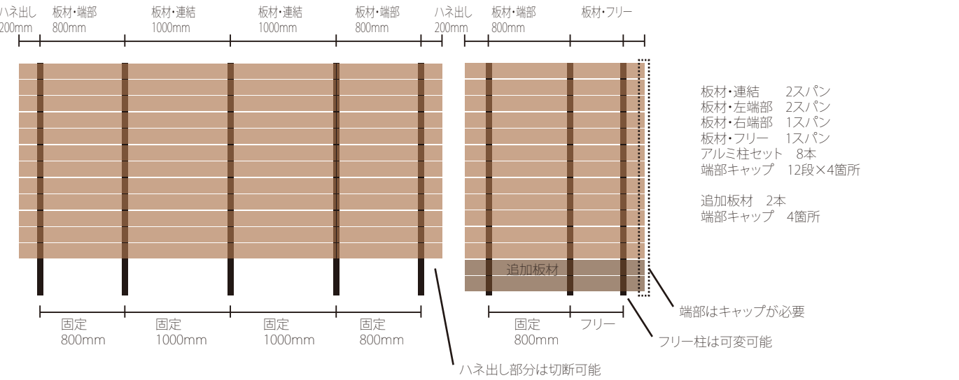
APF2212 L型の場合の計算方法
