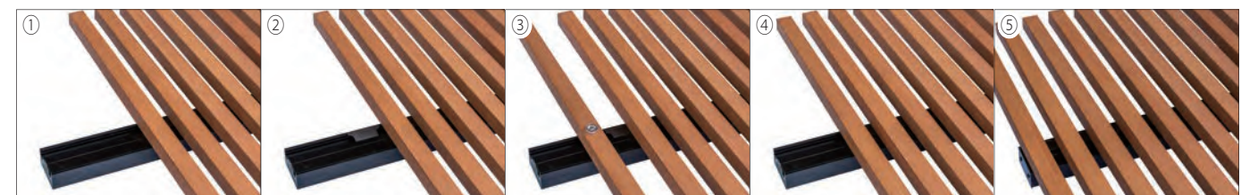
①アルミ横棧に格子の金具を引っ掛けます。 ②格子を留める金具をアルミ横棧に取り付けます。 ③格子の金具を取り付けた様子 ④順番に格子を取り付けます。 ⑤最後にストッパーを取り付けて完了です。
